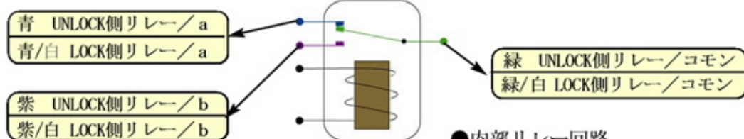
●内部リレー回路
