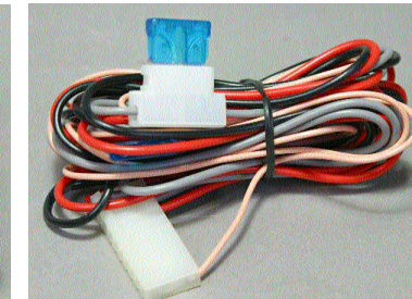
10ピンコネクター付 ハーネス
