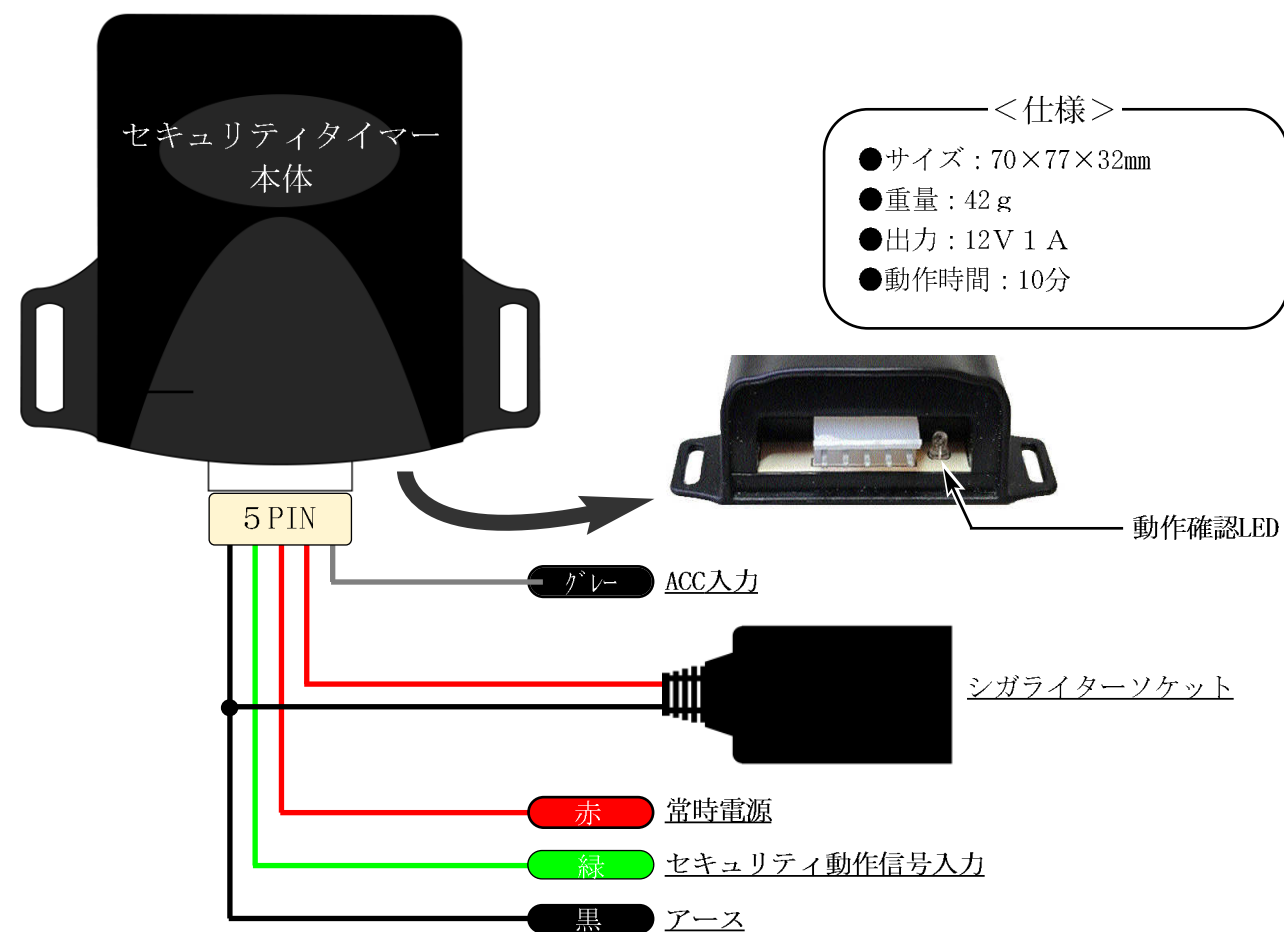
セキュリティタイマー接続概略
